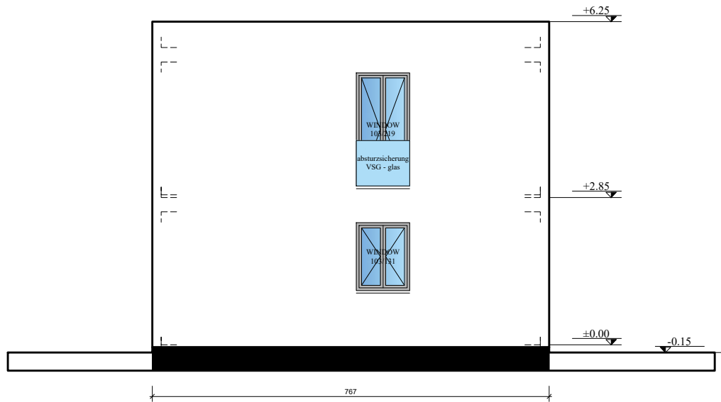
FASSADE A-B
