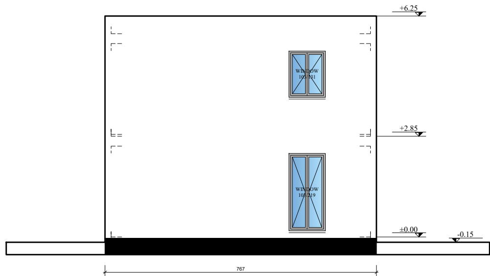
FASDADE B-A
