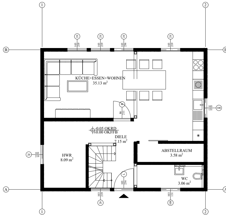
GEBÄUDEPLAN ±0.00 A = 68.42 m 2
