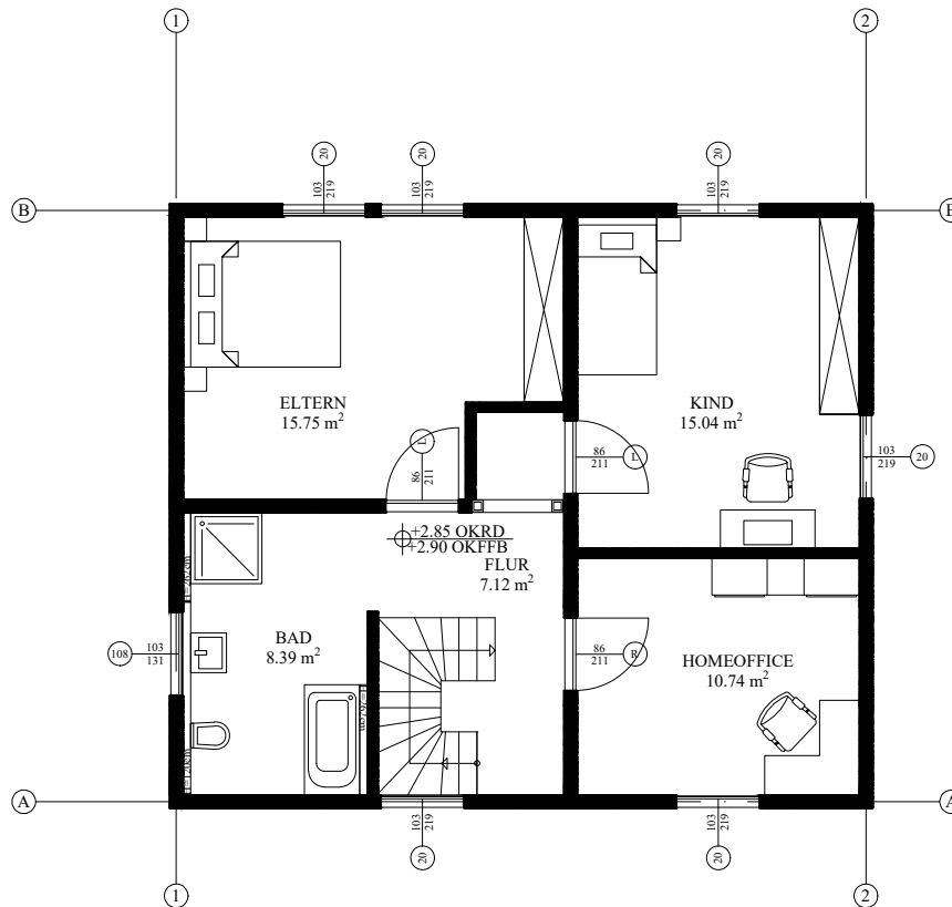
GEBÄUDEPLAN +2.90 A = 68.42 m 2
