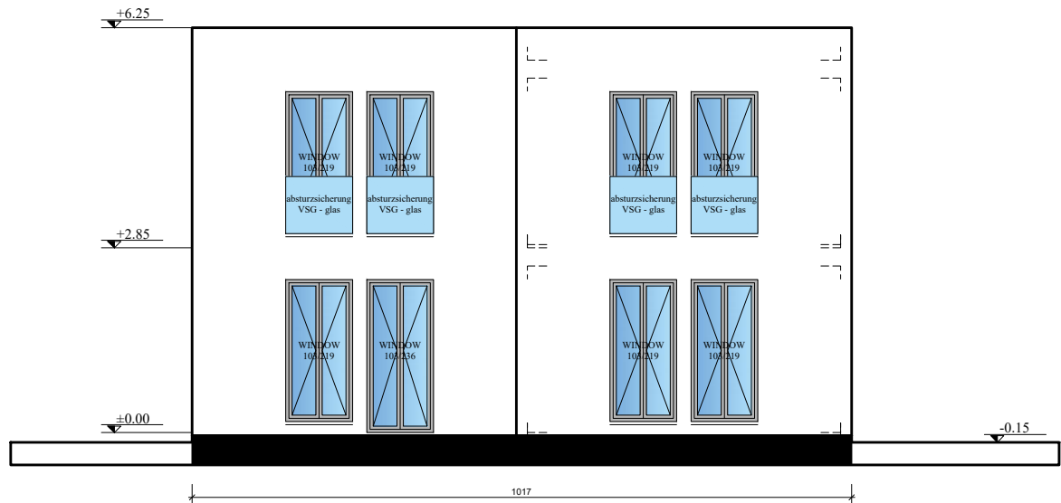
FASSADE A-B
