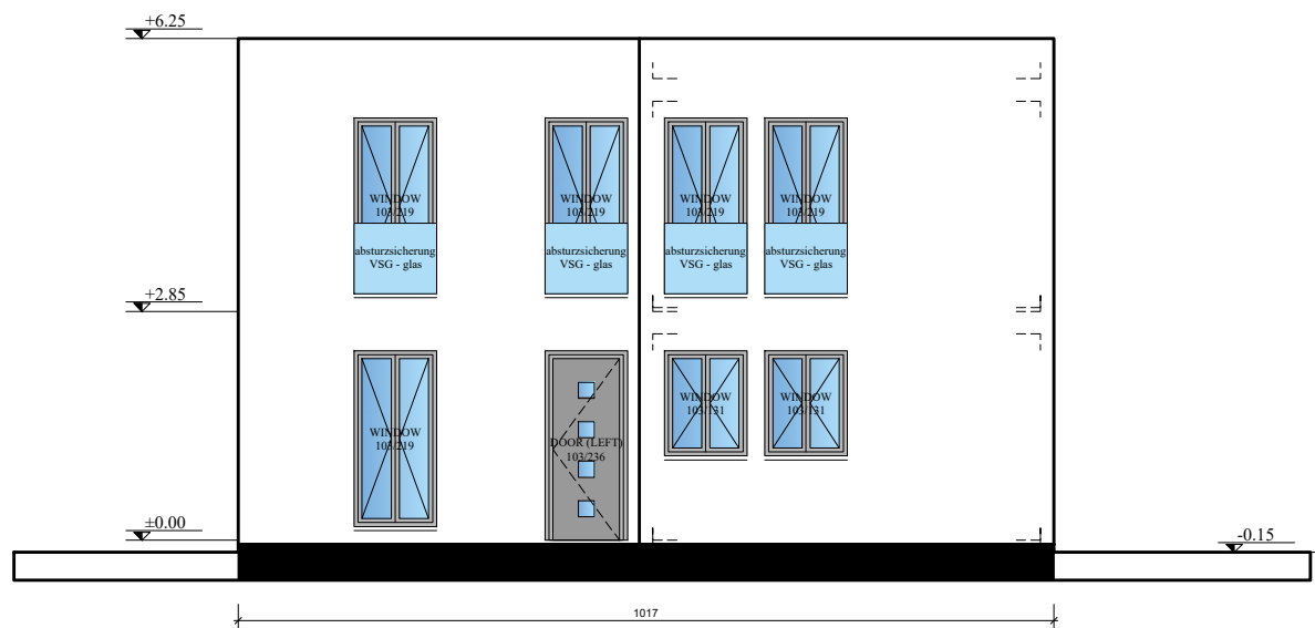
FASSADE B-A
