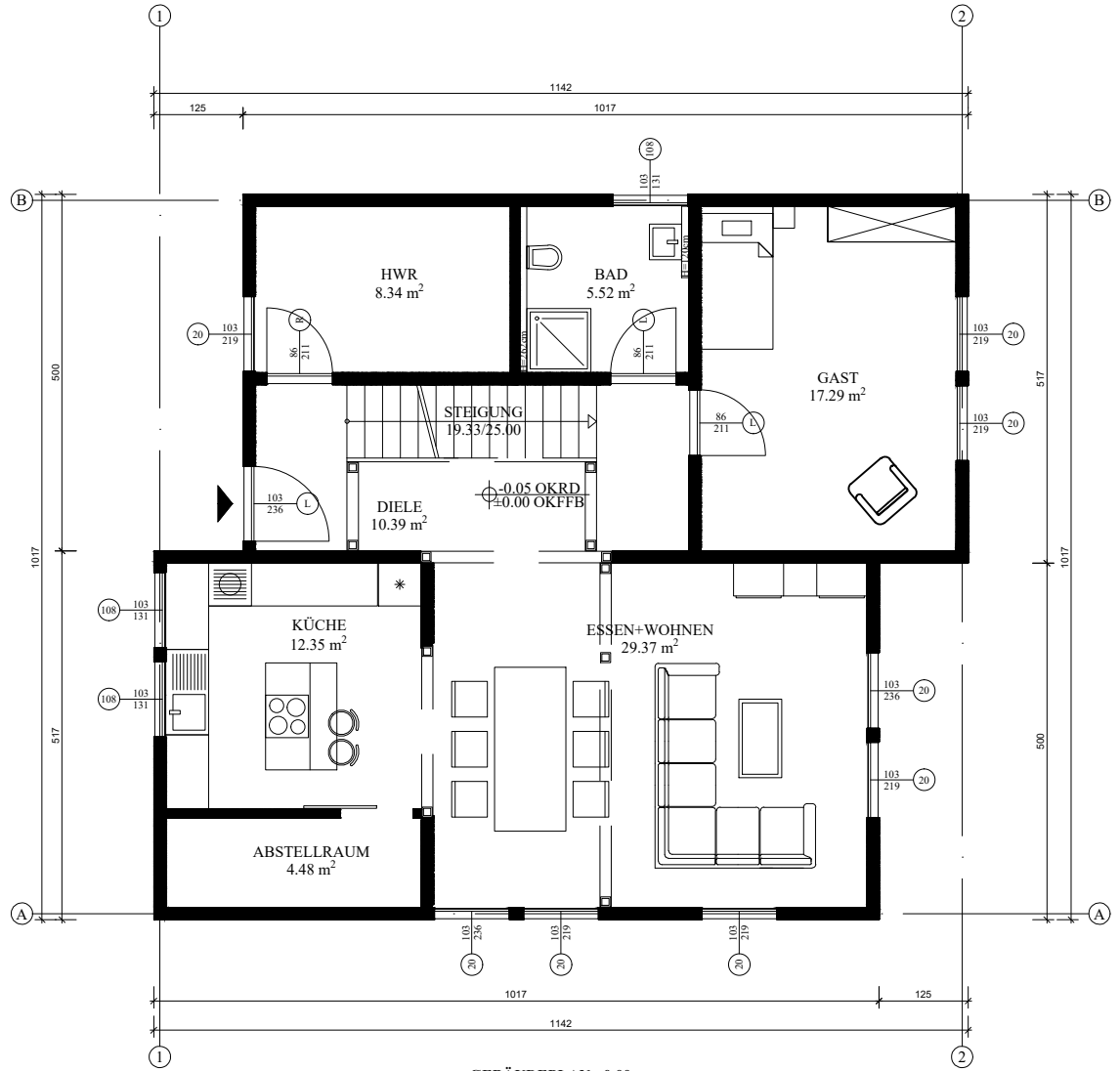
GEBÄUDEPLAN ±0.00 A = 103.64 m 2
