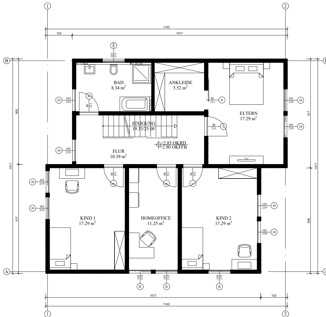
GEBÄUDEPLAN +2.90 A = 103.64 m 2
