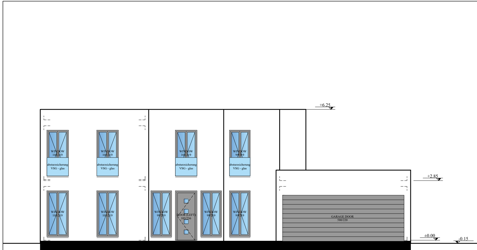
FASSADE 1-2
