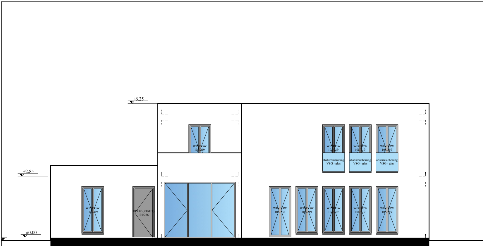
FASSADE 2-1
