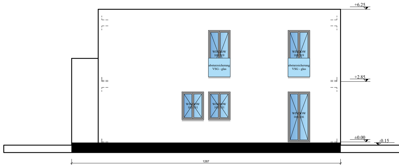
FASSADE B-A
