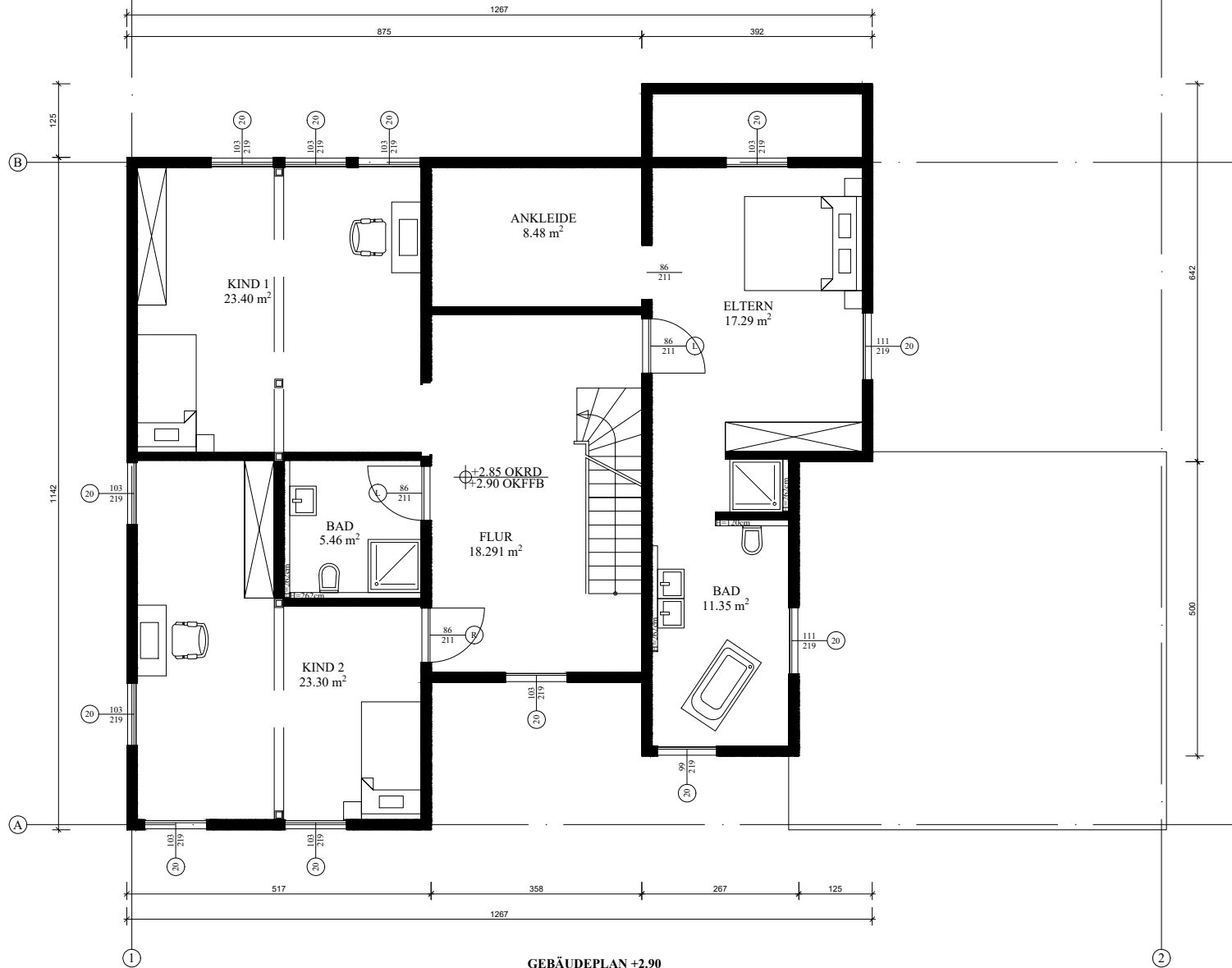
GEBÄUDEPLAN +2.90 A = 129.49 m 2
