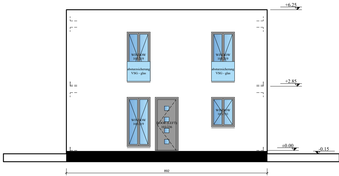
FASSADE 1-2
